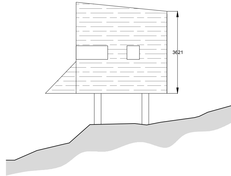
Elevation 3
