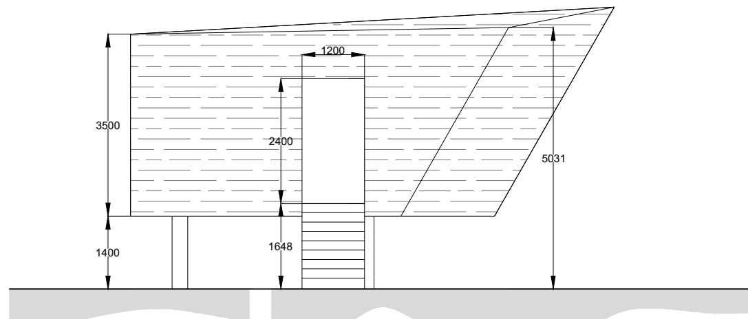
Elevation 1
